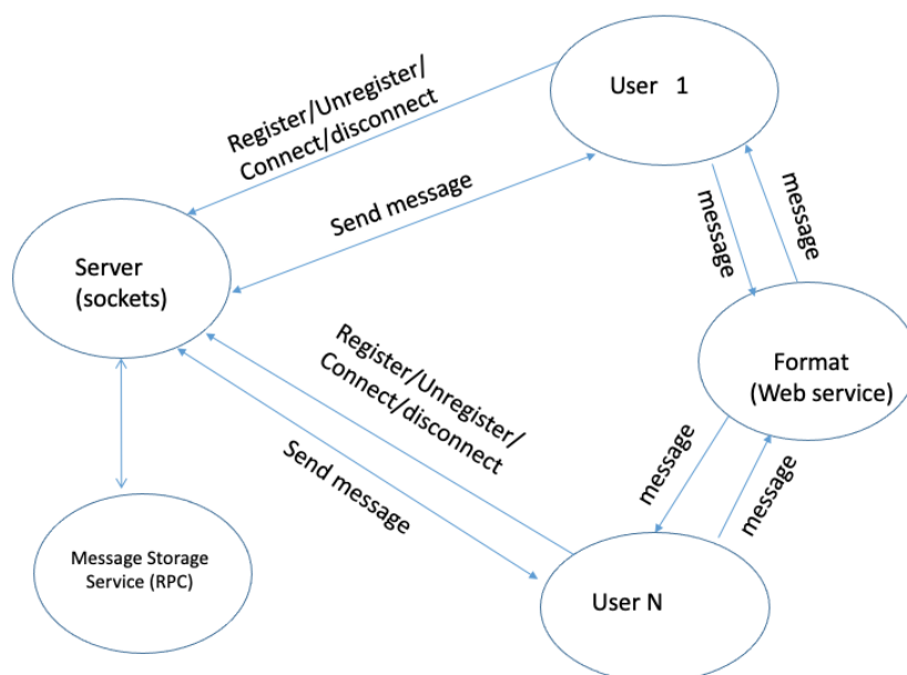
Figura 1: Servicio de notificación a desarrollar
